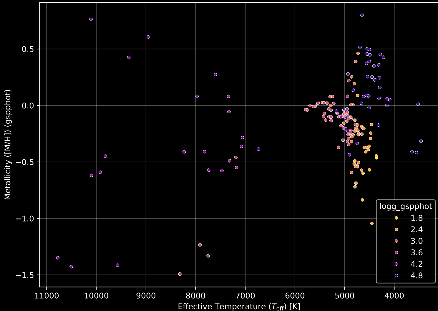
APOGEE DR17 Field: [195+18] Stellar Population Parameters (n= 173)
